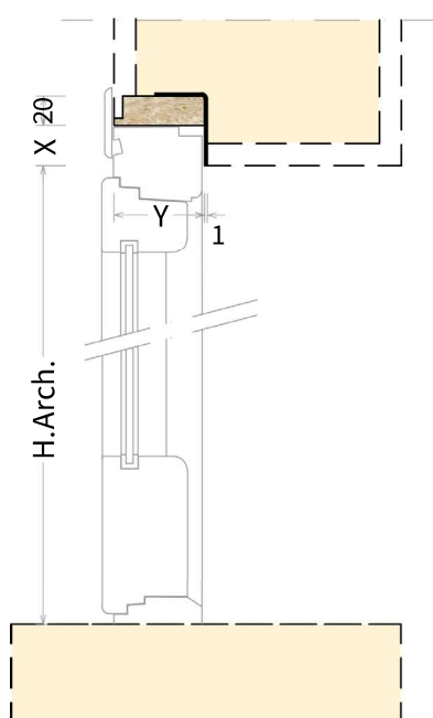
Profilo lamiera con X variabile
