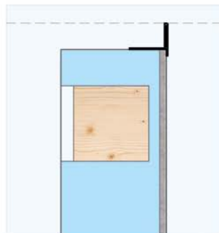
C Profilo parasigolo in pvc con retina. Idoneo per finitura muraria con intonaco esterno (con spessore di 15 mm).
