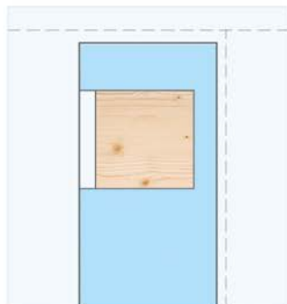
B Spalla priva di parasigolo e di fibrocemento dopo la guida. Finitura e spigolatura esterna a carico dell'impresa.
