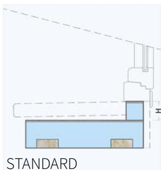
A Sottobancale con taglio termico per soluzione con serramento a filo muro interno. Costituito da base (64 mm) e listello sotto-serramento sfuso (44 m).
