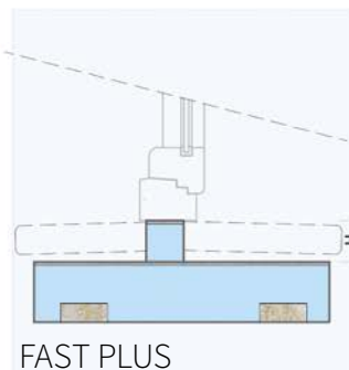
C Sottobancale con taglio termico per soluzione con serramento a metà mazzetta. Costituito da base e listello sotto-serramento.
