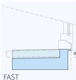
B Sottobancale per soluzione con serramento a filo muro interno. Costituito da base con listelli laterali e listello sotto-serramento. Idoneo anche per scossaline in alluminio.
