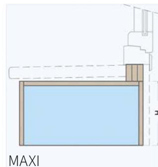
D Sottobancale Maxi per porta-finestra con funzione di fermagetto. Costituito da base in xps rivestito in duripanel e listello sotto-serramento.
