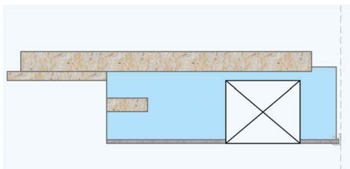
A Predisposizione superiormente sul soprabancale per l'alloggiamento del motore per sistemi di persiana automatizzata. Realizzazione a misura.
