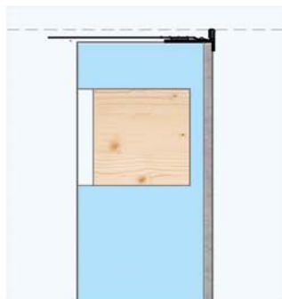
A Profilo parasigolo in pvc, con retina per favorire la realizzazione della rasatura muraria. Idoneo per finitura con termo-cannotto.
