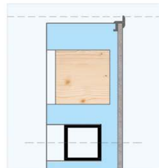
D Tubolare in acciaio (40x40 mm) con relative zanche a murare, integrato su spalle termiche. Funzionale al fissaggio di inferriate e/o paranebbi.
