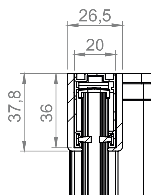
SEZ. VERTICALE
