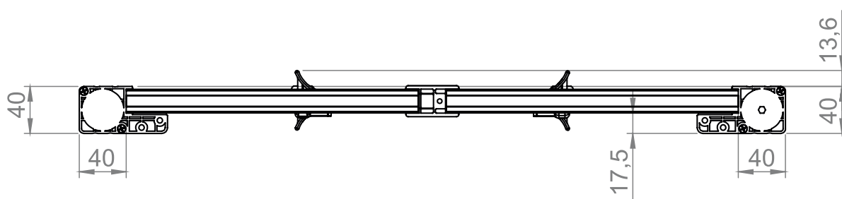
SEZ. ORIZZONTALE
