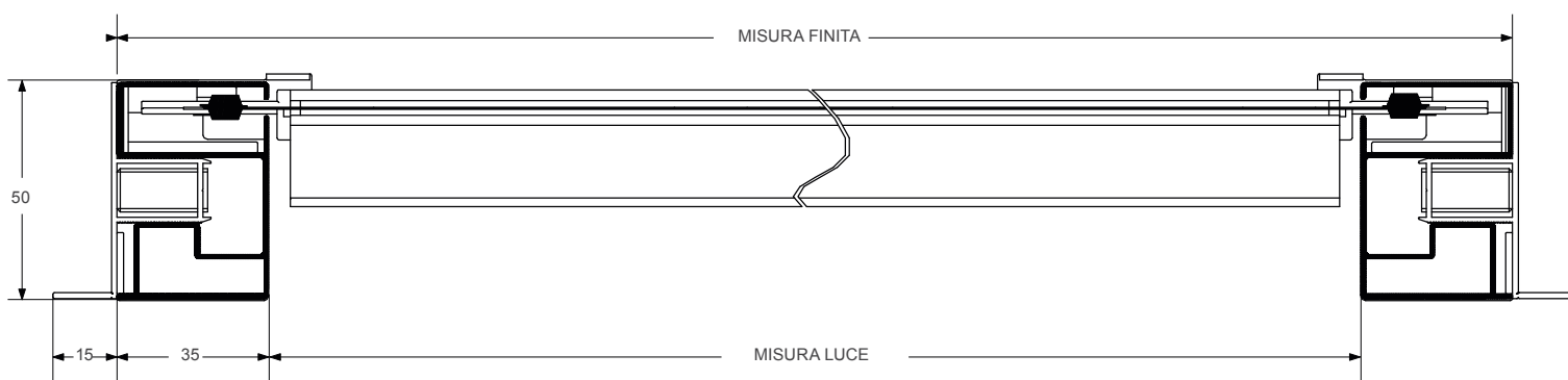
SEZ. ORIZZONTALE
