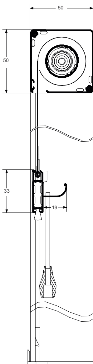
SEZ. VERTICALE
