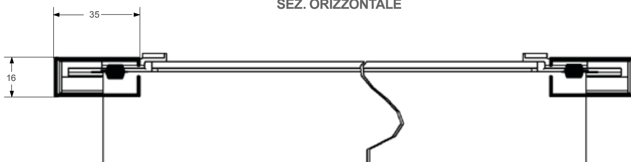
SEZ. ORIZZONTALE
