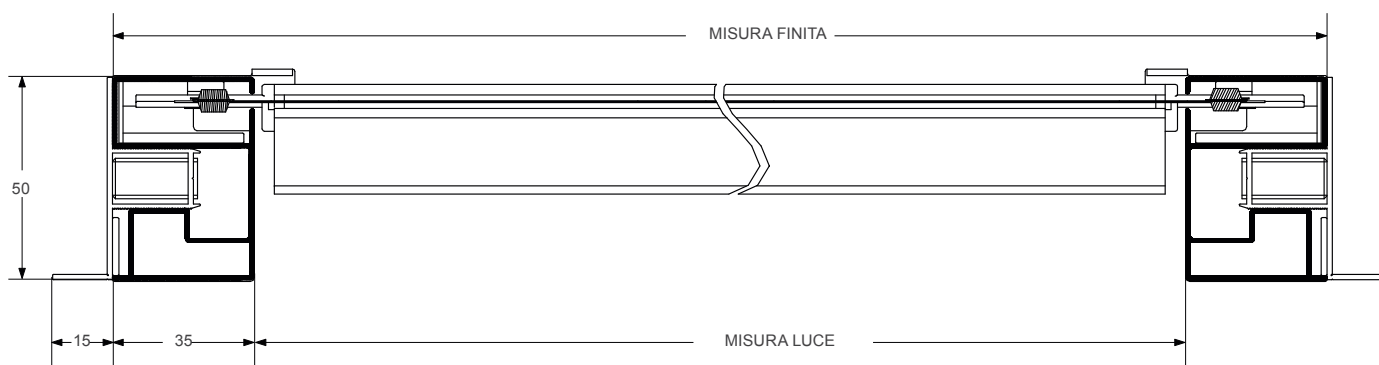
SEZ. ORIZZONTALE
