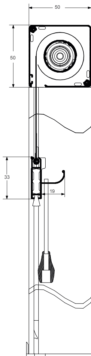
SEZ. VERTICALE
