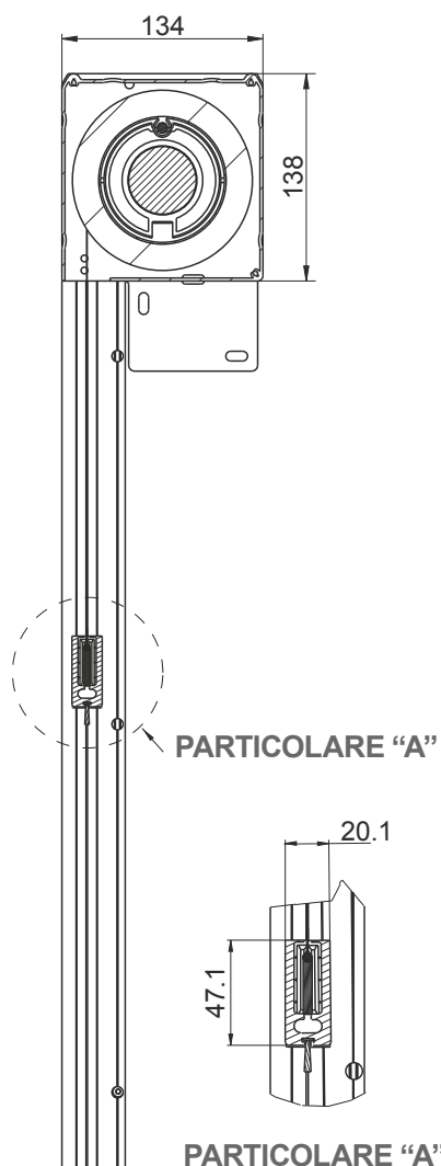
SEZ. VERTICALE
