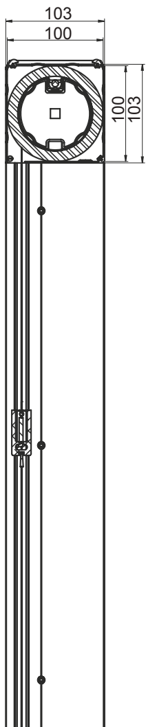
SEZ. VERTICALE
