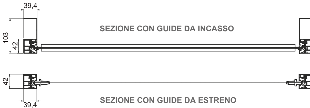
SEZ. ORIZZONTALE
