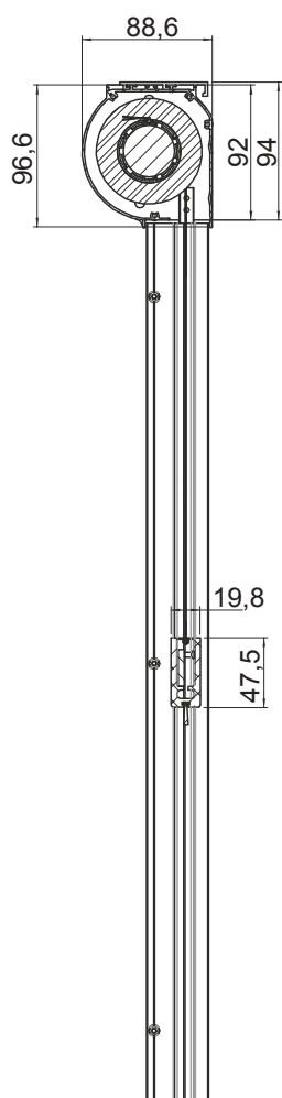
SEZ. VERTICALE
