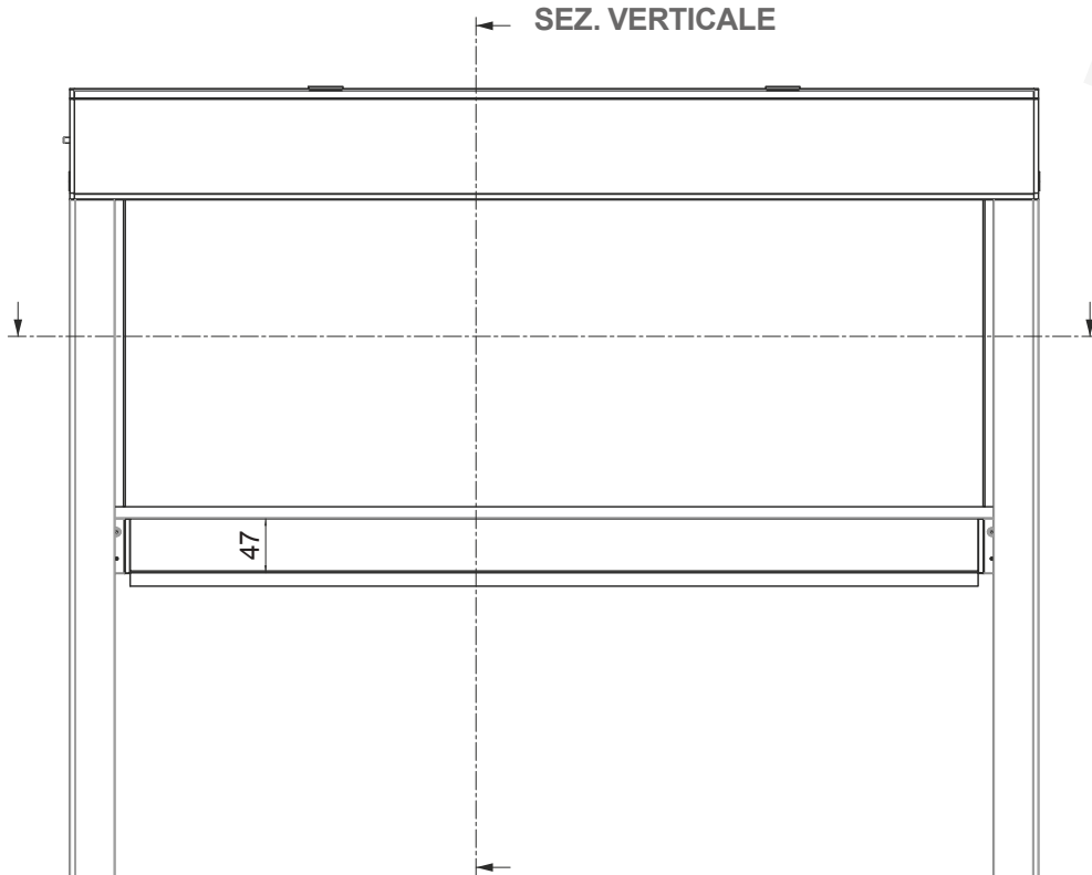
SEZ. VERTICALE
