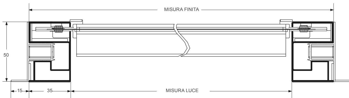
SEZ. ORIZZONTALE
