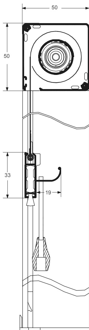
SEZ. VERTICALE
