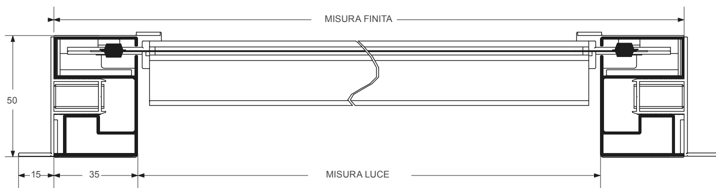
SEZ. ORIZZONTALE
