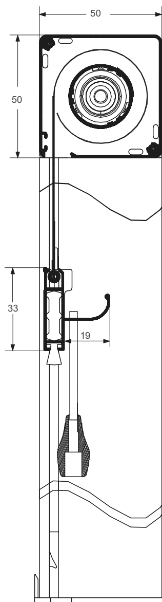
SEZ. VERTICALE
