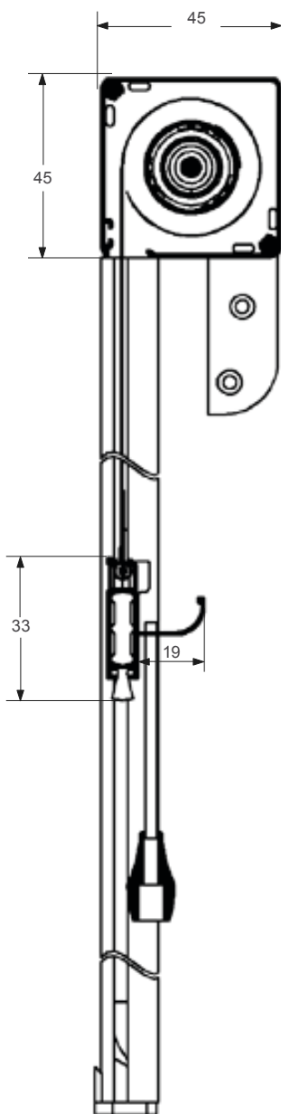
SEZ. VERTICALE
