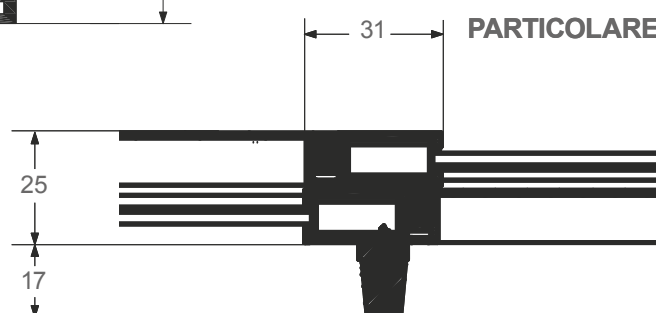
SEZ. ORIZZONTALE
