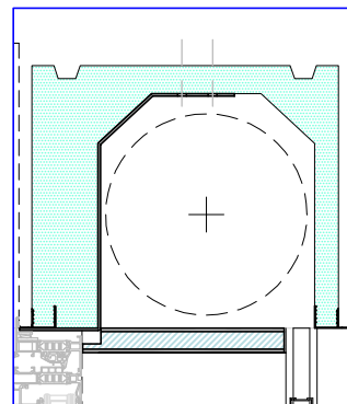
Staffa di rinforzo in lamiera zincata per fissaggio serramento a solaio * disponibile SOLO con Cassonetti CSP35
