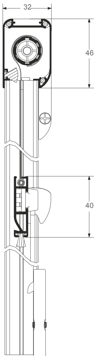
SEZ. VERTICALE
