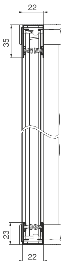
SEZ. VERTICALE
