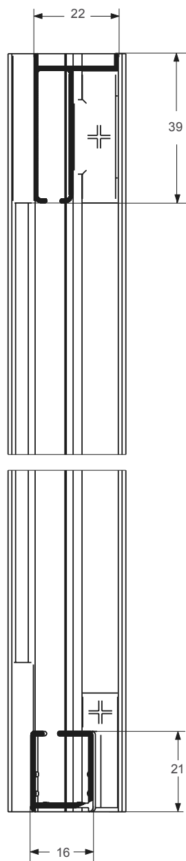
SEZ. VERTICALE
