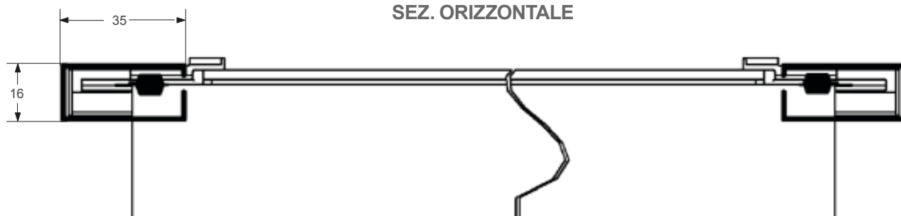
SEZ. ORIZZONTALE
