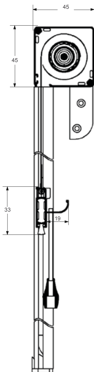
SEZ. VERTICALE
