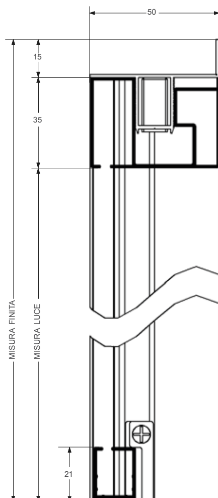
SEZ. VERTICALE
