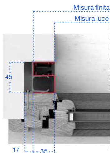
Sezione orizzontale
