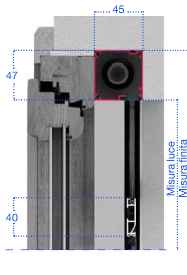
Sezione verticale
