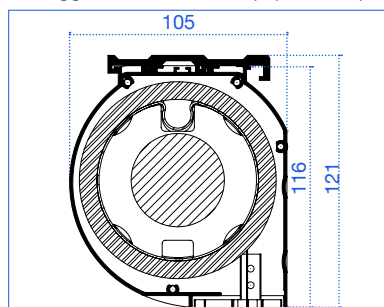
Fissaggio a soffitto con clip (standard)
