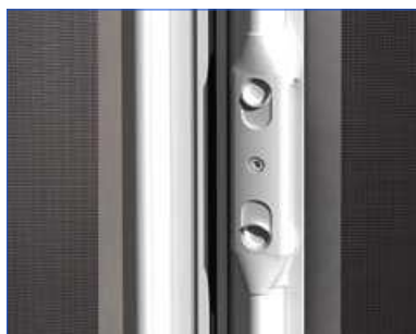
Chiusura con cricchetto per il due ante
