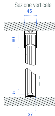
Maniglia per incasso (solo su versione ad incasso se specificato sull'ordine)
