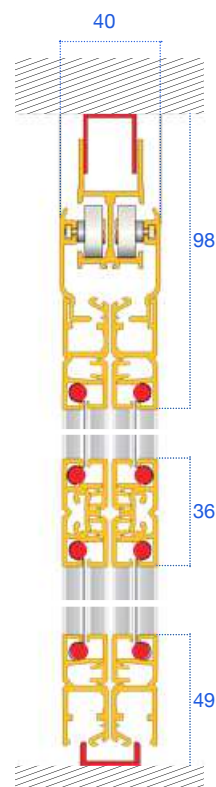
Sezione verticale
