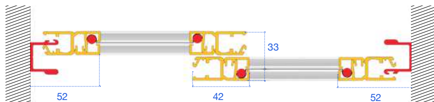
Sezione orizzontale
